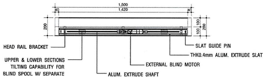
③ EVB 외부차양 평면상세도
