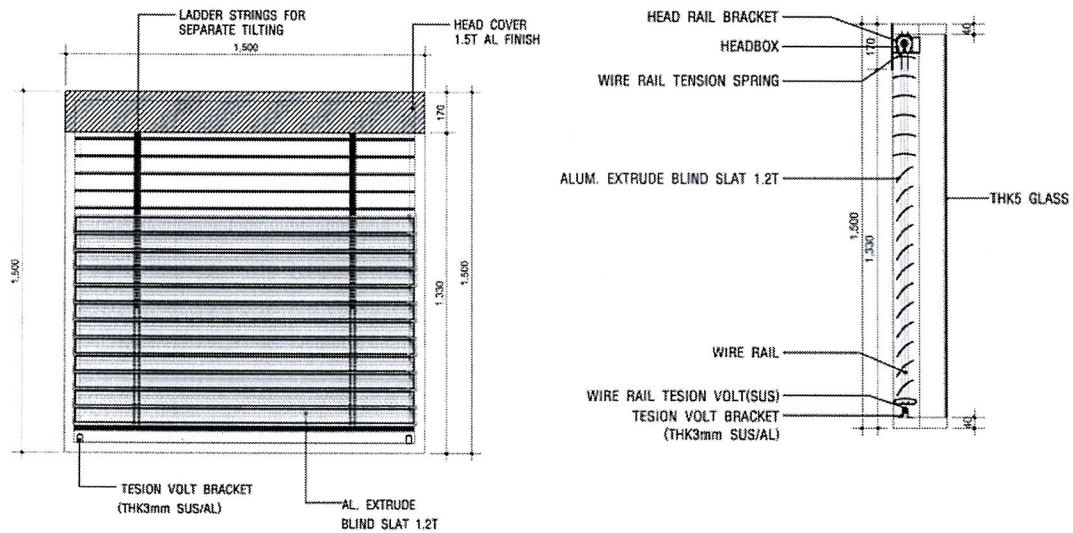
② EVB 외부차양 단면상세도
