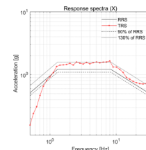
내진성능 실험
