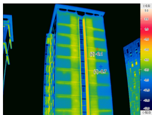
내단열 적용 건물의 열화상 촬영 결과
