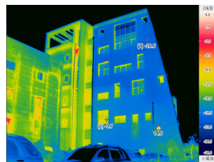
외단열 적용 건물의 열화상 촬영 결과
