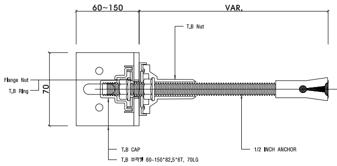
단면도
