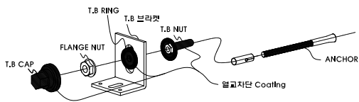
분해도
