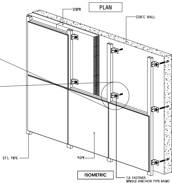
그림 3: 싱글앵커타입 베이직 프레임용 설치도
