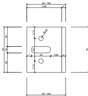
측면도
