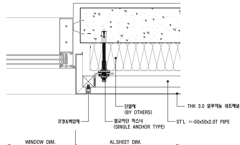
03 창호 주변 평면 상세도
