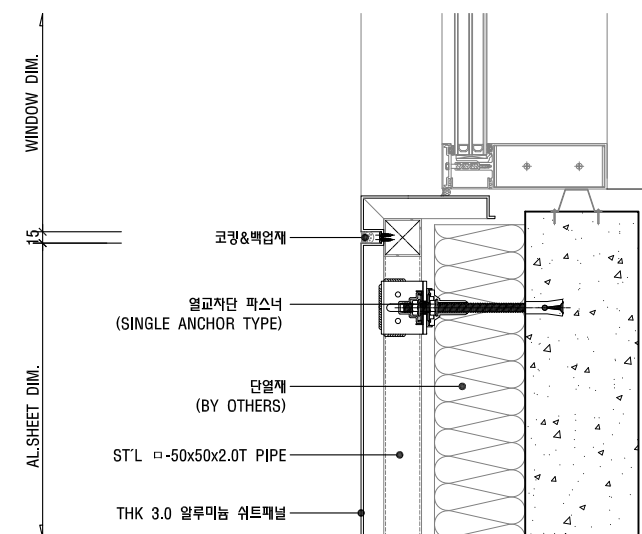
06 창호 상부 단면 상세도
