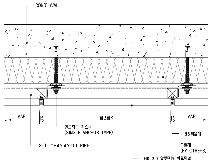
01 기준 평면 상세도
