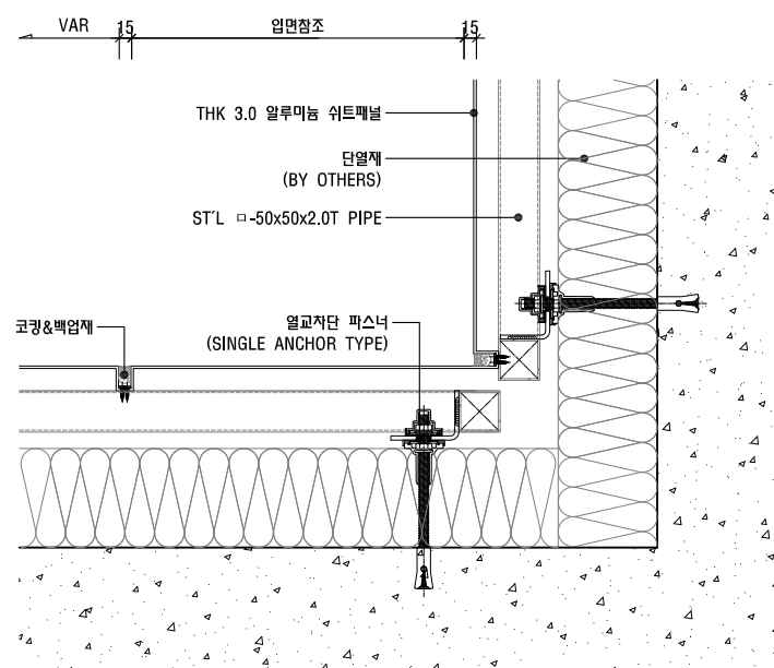
04 코너 평면 상세도 - OUTCONER
