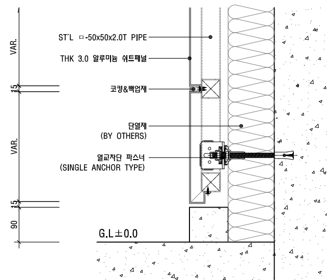
08 하부 단면 상세도
