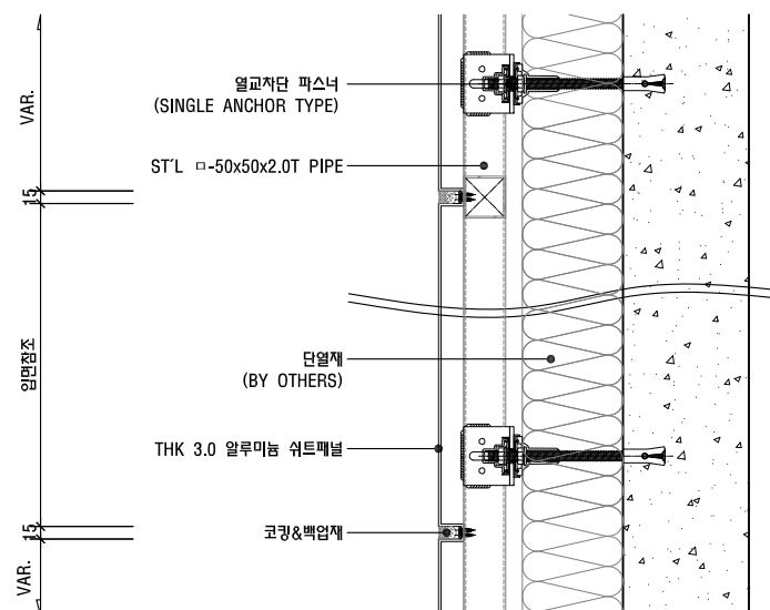
05 기준 단면 상세도
